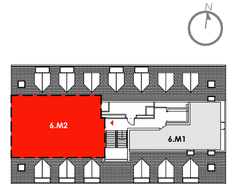
SCHEMAT KONDYGNACJI
