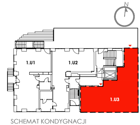
SCHEMAT KONDYGNACJI
