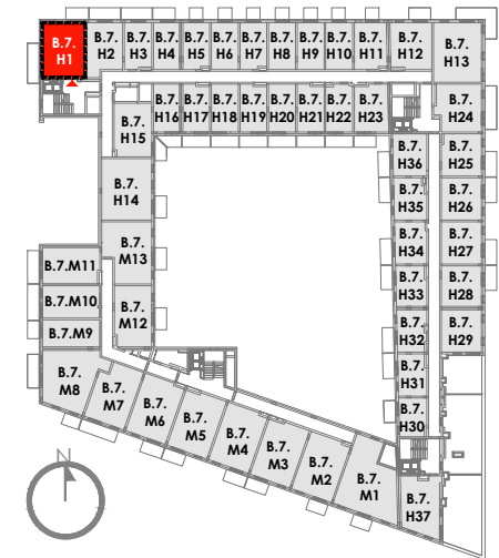
SCHEMAT KONDYGNACJI
