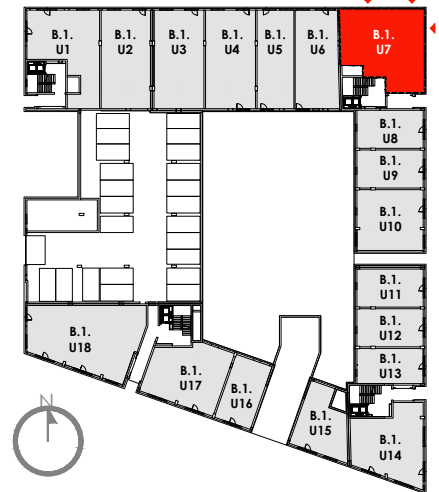
SCHEMAT KONDYGNACJI
