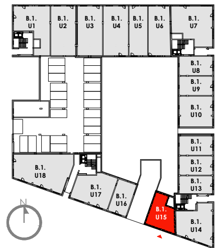
SCHEMAT KONDYGNACJI
